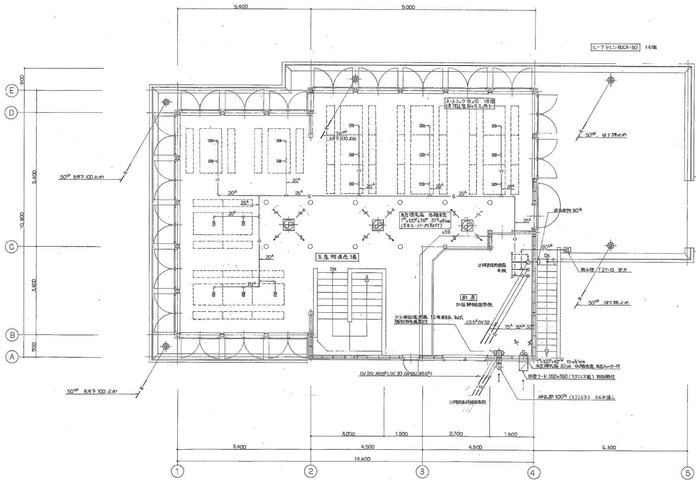
2階平面図 5-1/50
